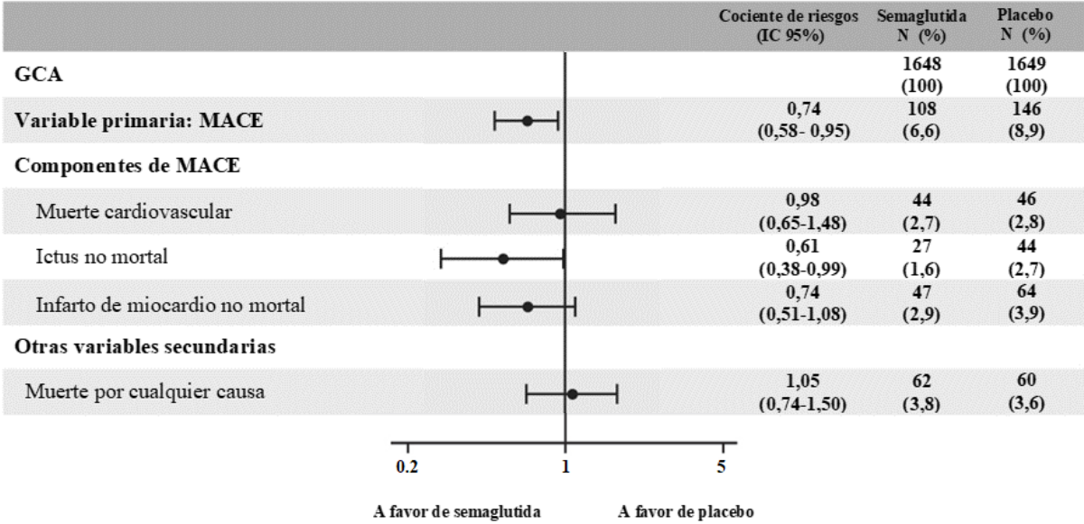
Figura 4 Diagrama de bosque: análisis del tiempo transcurrido hasta la primera aparición de la variable compuesta, sus componentes y muerte por cualquier causa (SUSTAIN 6)
