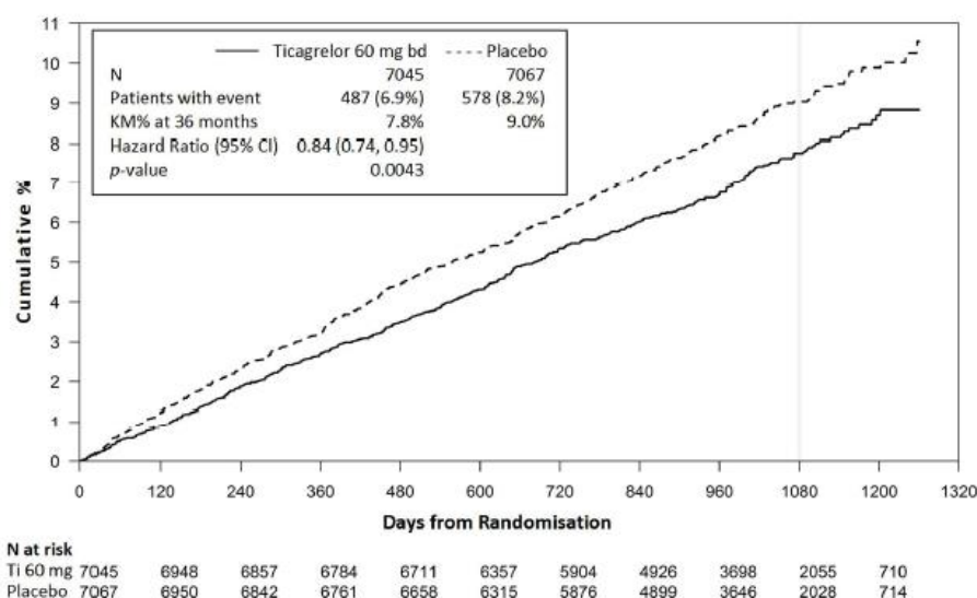
Figura 2 - Análisis de la variable principal de valoración clínica combinada de muerte CV, IM e ictus (PEGASUS)
